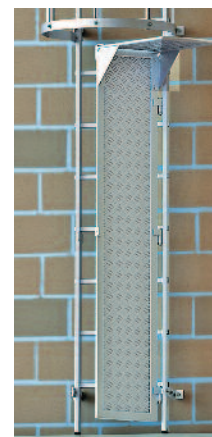
Steigschutztüre mit Deckel
