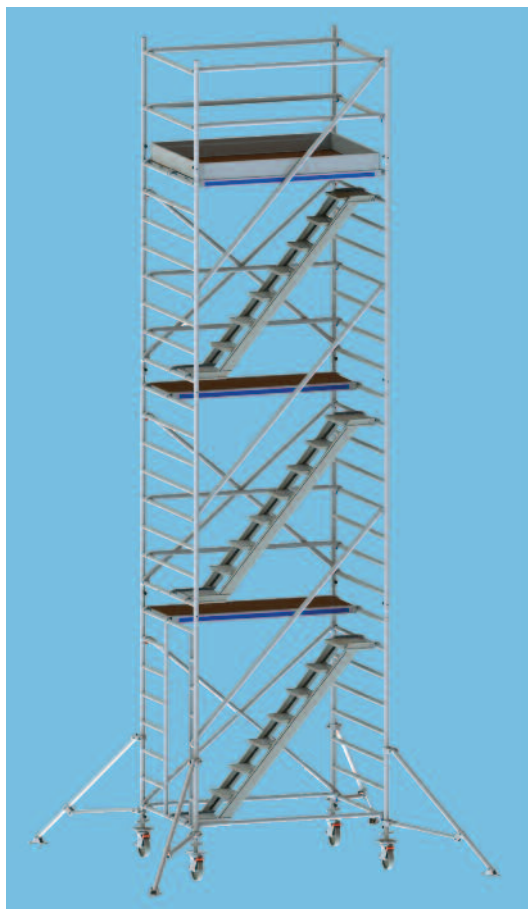
Art. Nr. 733064 / 743064
