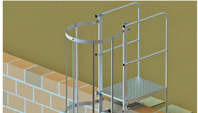
Ausstieg mit Übergang
