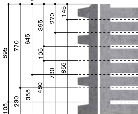
Schnittmöglichkeiten
