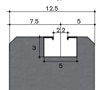
Jordalschiene Typ AEPPLI
