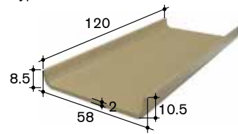
Typ G-258
