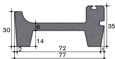
Typ 30.4 Jungvieh
