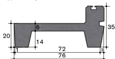
Typ 20.4 Jungvieh
