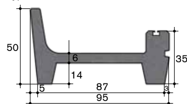
Typ 50.4 Grossvieh
