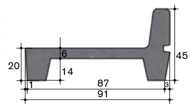
Typ 20.4 Grossvieh
