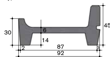
Typ 30.4 Grossvieh
