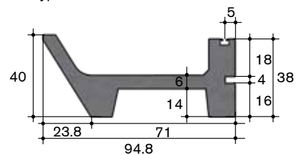
Typ 6bj AEPPLI Grossvieh
