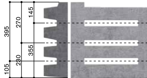
Schnittmöglichkeiten
