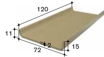
Typ G-242
