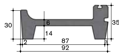
Typ 30.4 Grossvieh
