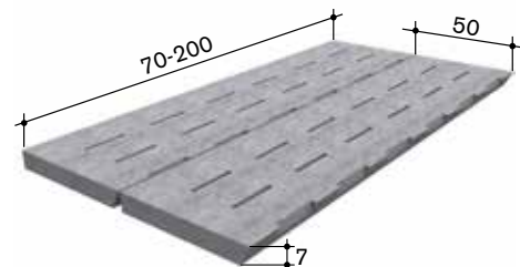
Typ 17/05 mit 5% Durchlass
