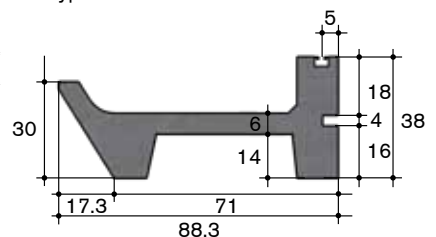
Typ 6cj AEPPLI Grossvieh
