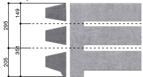
Schnittmöglichkeiten
