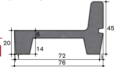
Typ 20.4 Jungvieh
