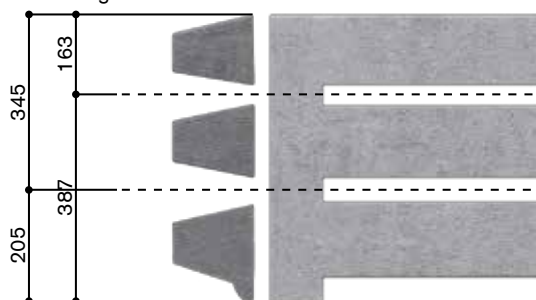
Schnittmöglichkeiten
