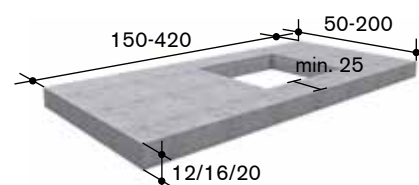
Schonlau Gussroste
