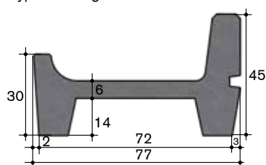
Typ 20 Jungvieh
