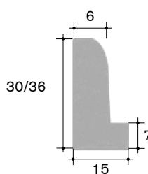
Lochmasse Für 30cm/36cm Höhe
