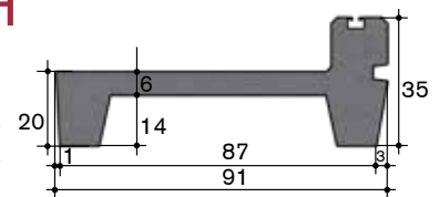
Typ 20.4 Grossvieh
