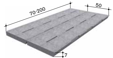
Typ 17/02 mit 2% Durchlass
