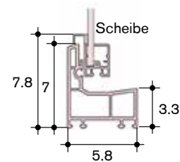
Querschnitt Fenster
