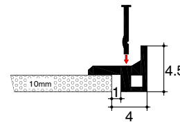
Gummi-Winkelprofil
