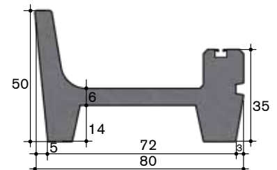
Typ 50.4 Jungvieh
