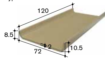
Typ G-272
