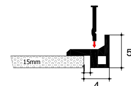
Gummi-Winkelprofil
