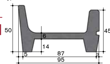
Typ 50.4 Grossvieh
