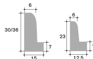
Lochmasse Für 30cm/36cm Höhe
