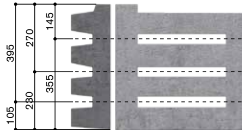
Schnittmöglichkeiten 35mm
