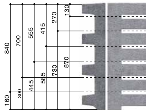
Schnittmöglichkeiten
