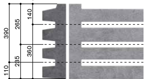
Schnittmöglichkeiten 30mm
